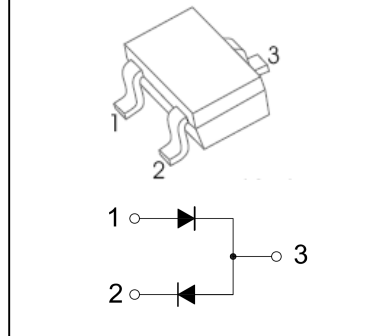
SOT-323
